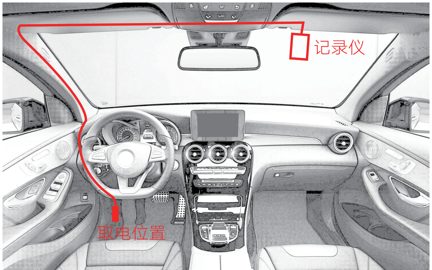
记录仪安装取电走线示意图
